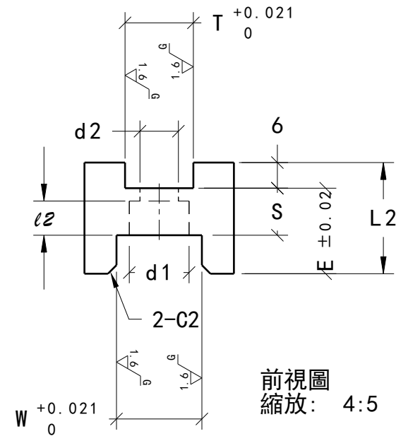
前視圖 縮放: 4:5
