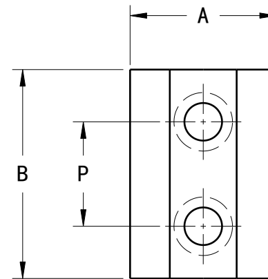
前視圖 縮放: 4:5
