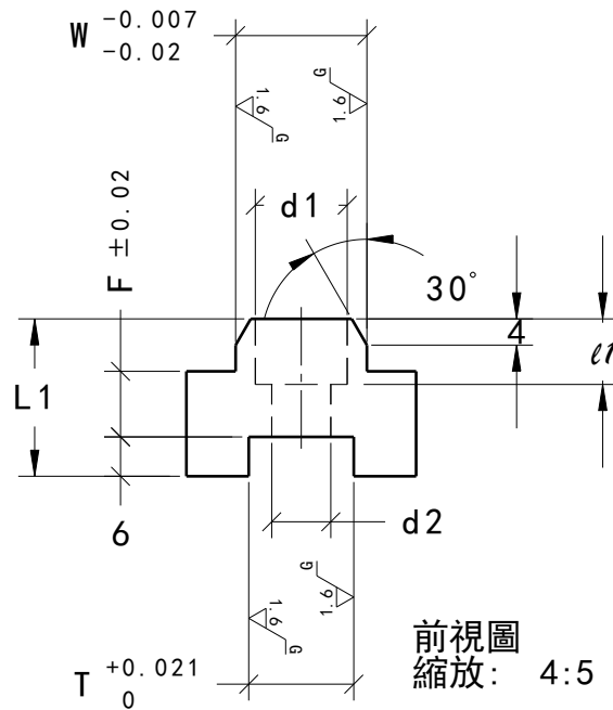
前視圖 縮放: 4:5
