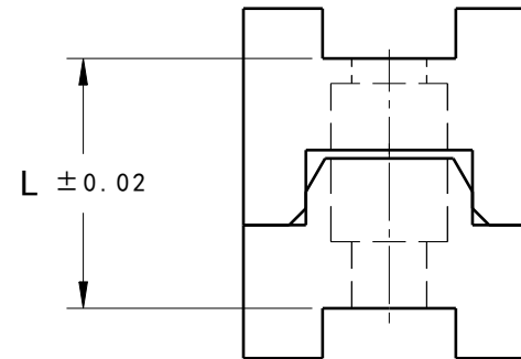
前視圖 縮放: 1:1
