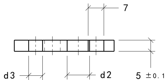
剖面視圖B-B 縮放: 1:1
