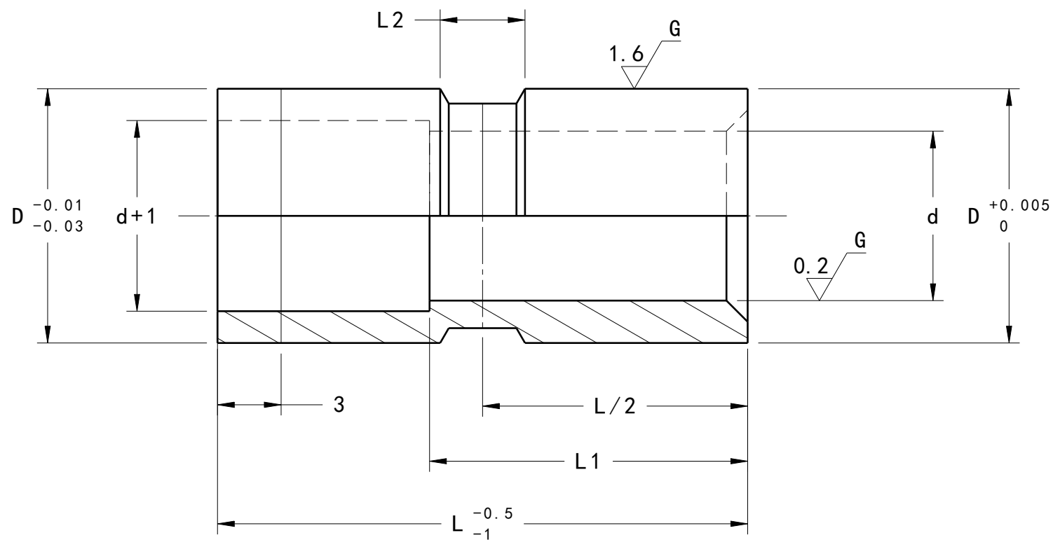
剖面視圖A-A 縮放: 4:1
