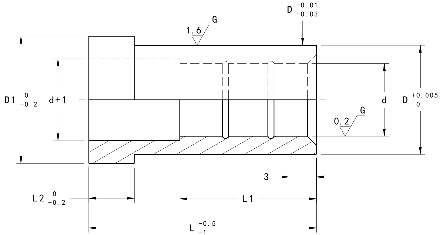
剖面視圖A-A 縮放: 4:1
