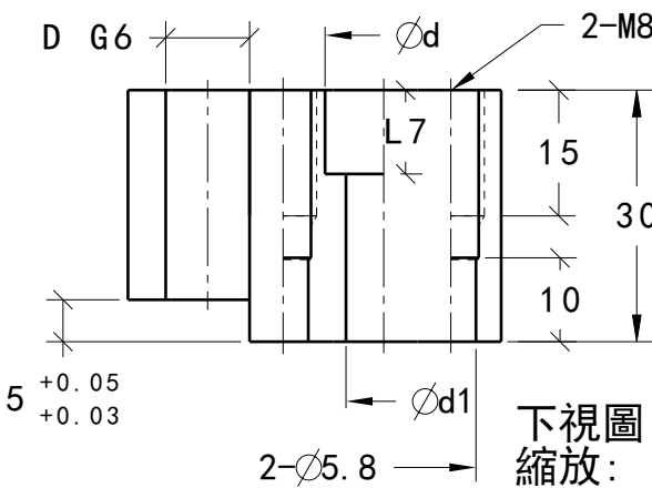
前視圖 縮放: 1:1
