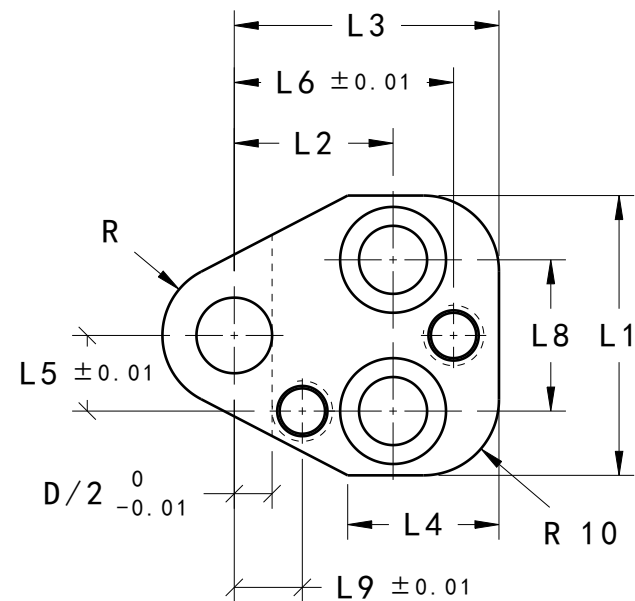
前視圖 縮放: 1:1
