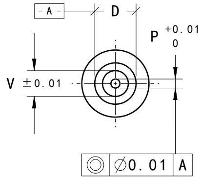
右視圖 縮放: 7:1
