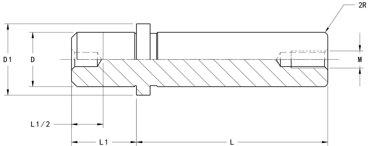
Section view A-A Scale: 6:5
