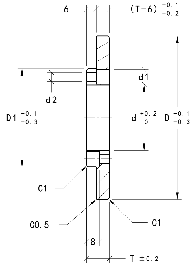
剖面視圖A-A 縮放: 3:4
