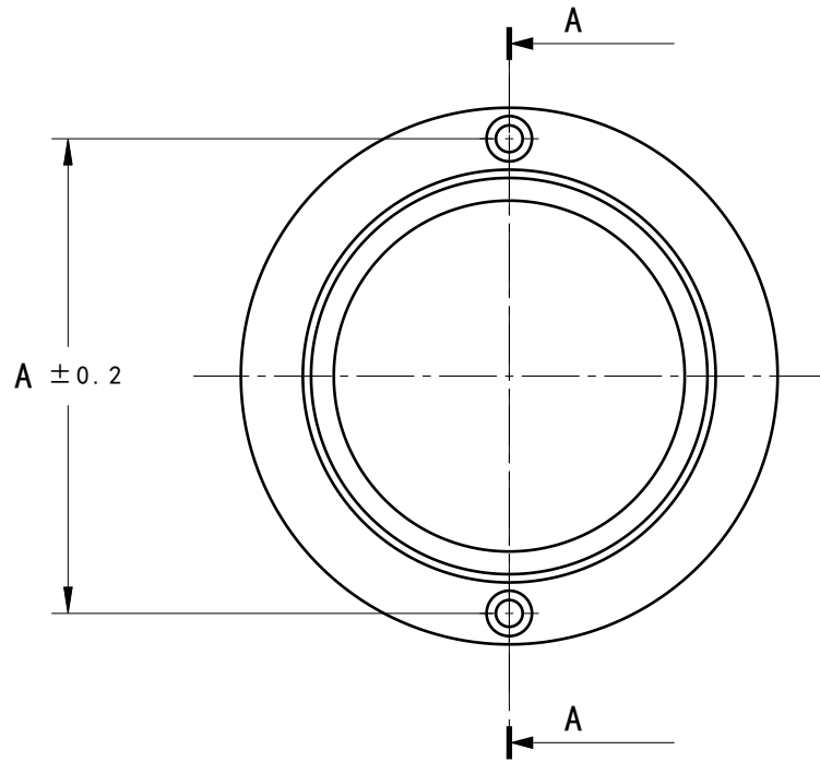
前視圖 縮放: 1:2
