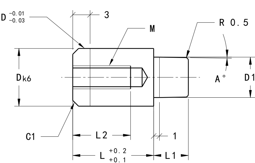
剖面視圖B-B 縮放: 5:2
