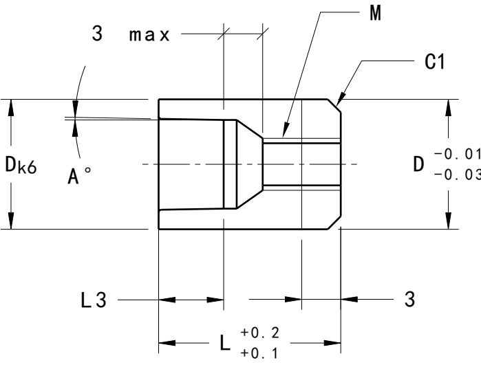
剖面視圖C-C 縮放: 5:2
