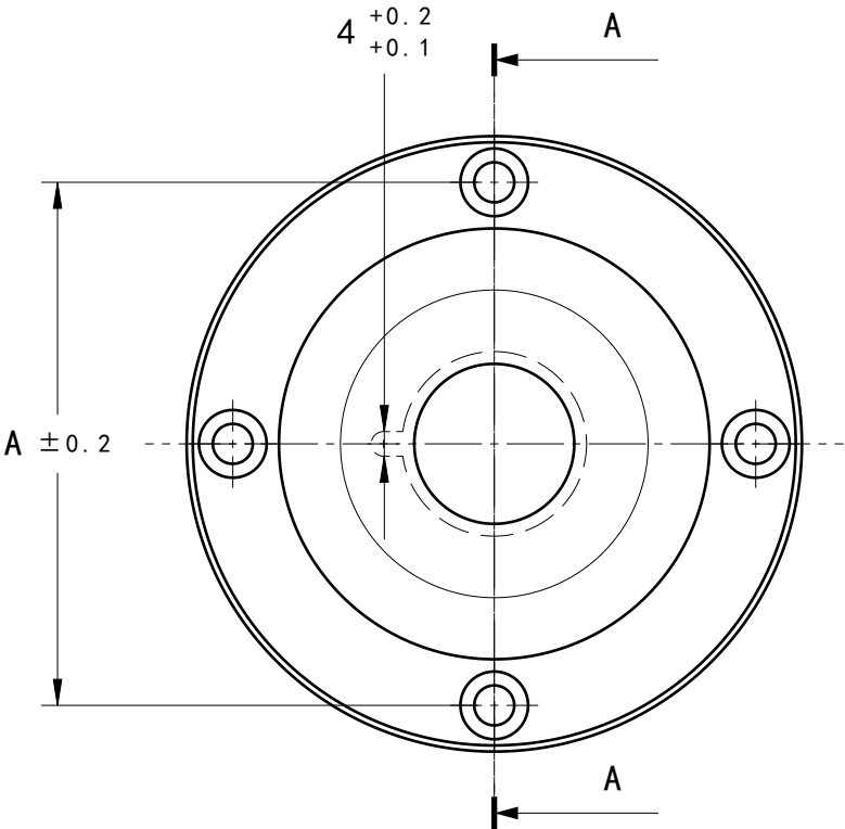
前視圖 縮放: 3:4
