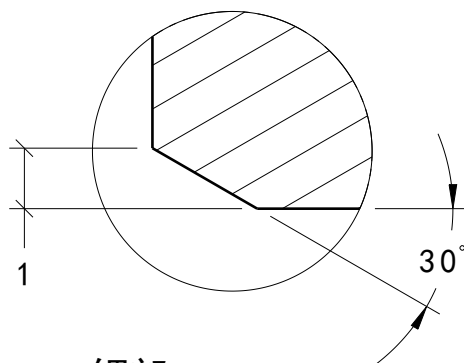
細部 B 縮放: 8:1
