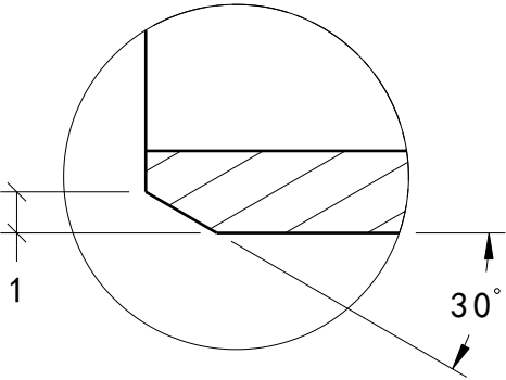
細部 B 縮放: 5:1
