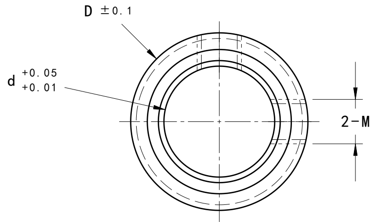
Left view Scale: 3:1
