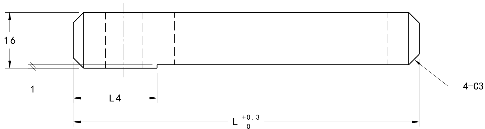
下視圖 縮放: 3:2
